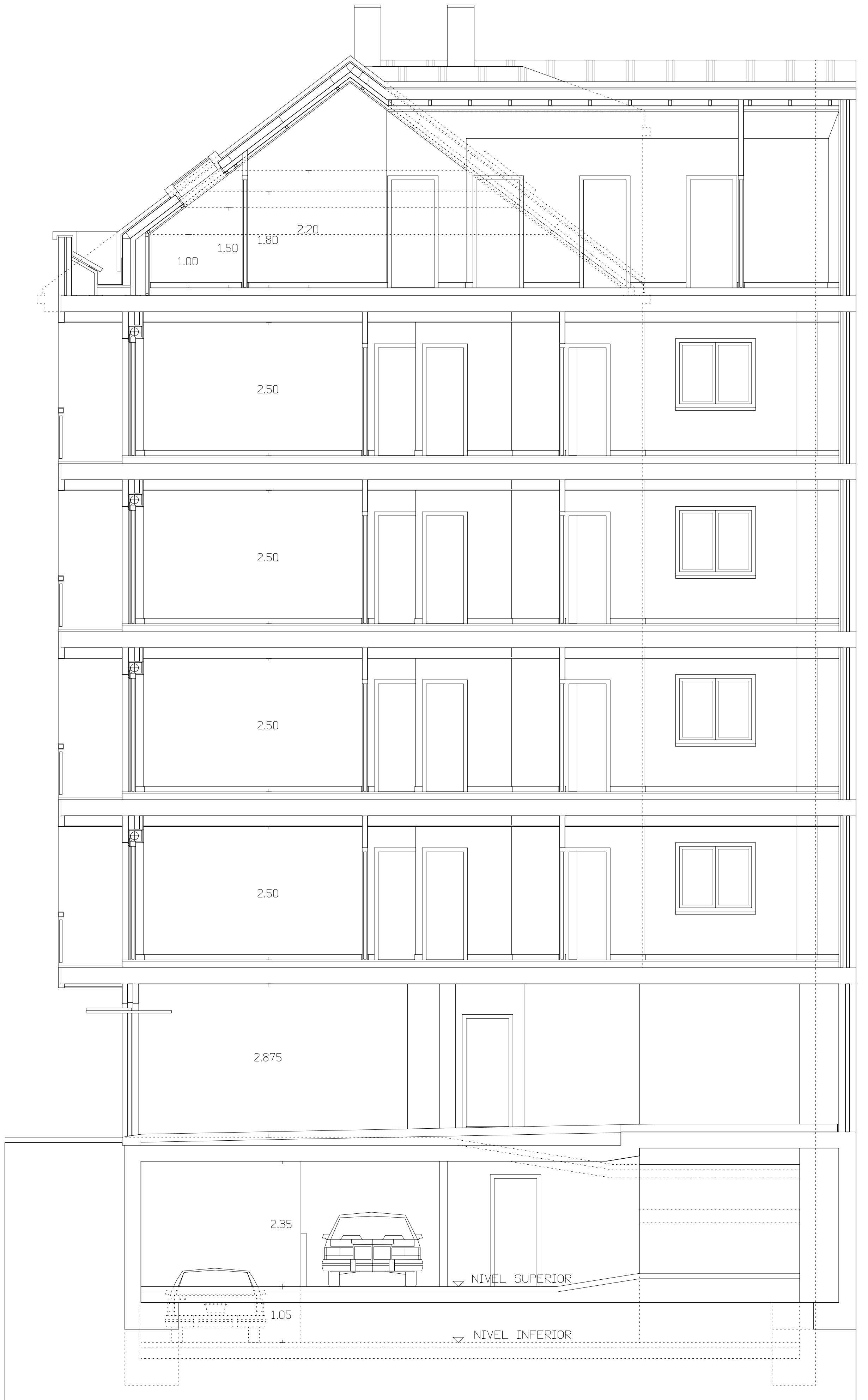
SECCION TRANSVERSAL T2-T2
