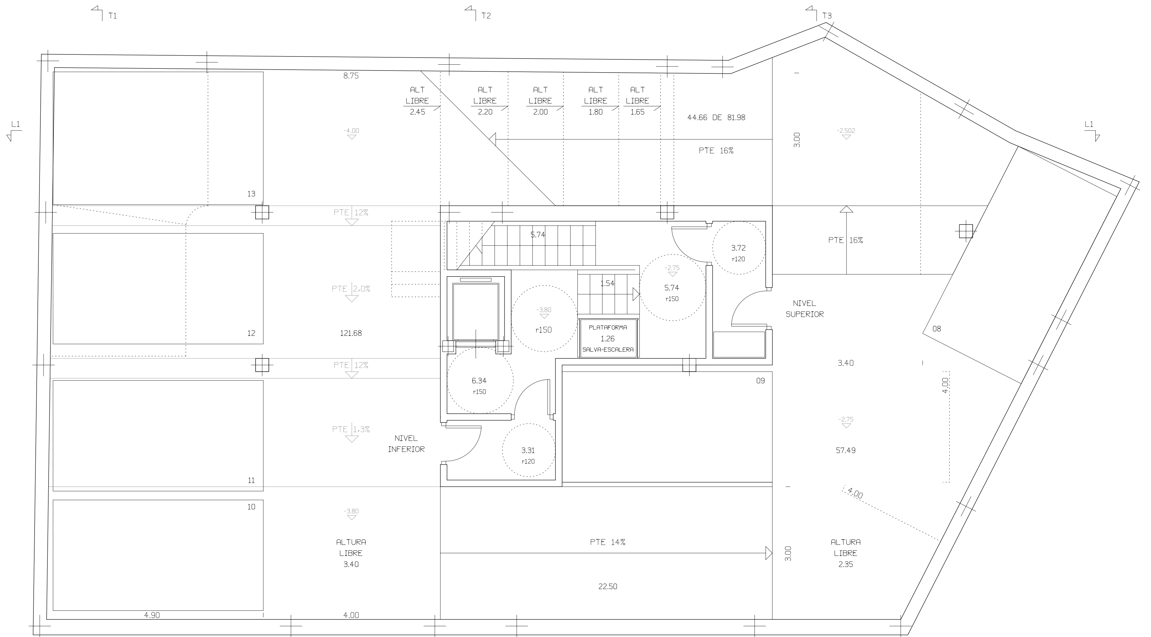
PLANTA SOTANO
