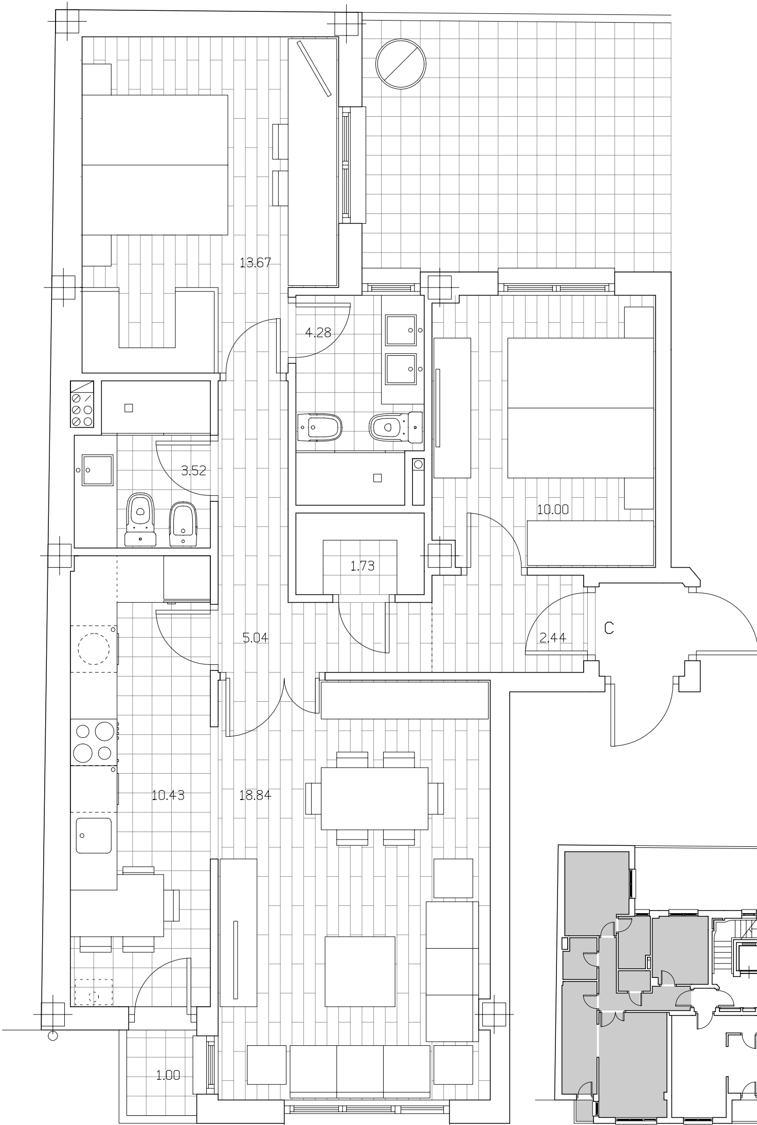
VIVIENDA "TIPO C" EN PLANTAS 3/4
