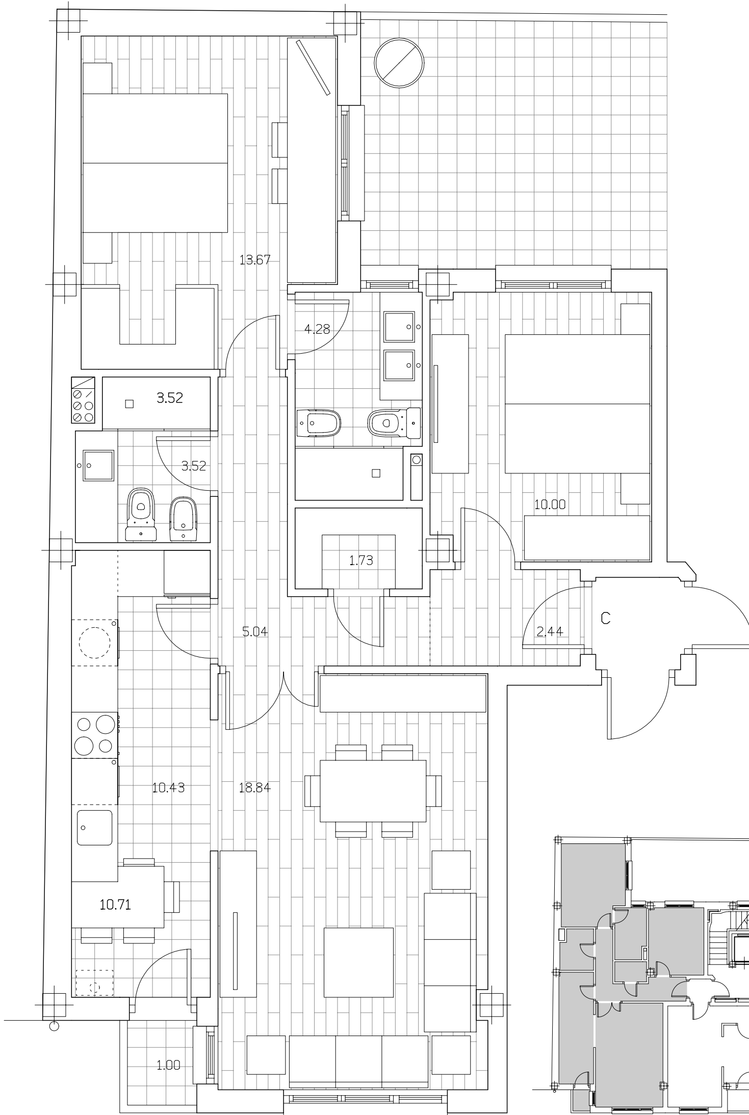
VIVIENDA "TIPO C" EN PLANTAS 1/2
